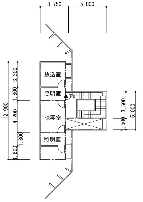
川内文化ホール3階平面図S=1:300
